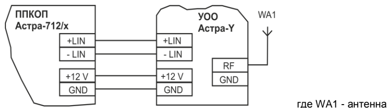
Рисунок 7 - Схема подключения ППКОП
