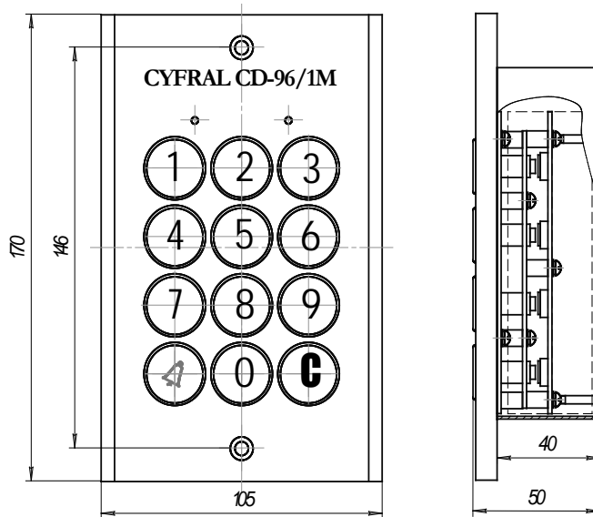
Рисунок А.2 Габаритные и установочные размеры панели кодовой ЦИФРАЛ CD-96/1M
