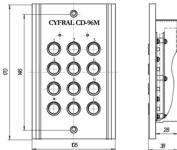
Рисунок А.1 Габаритные и установочные размеры панели кодовой ЦИФРАЛ CD-96M
