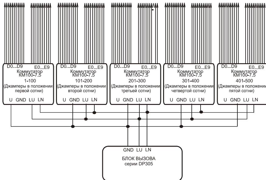
Рис.1 Вариант схемы подключения трех КМ100-7.5 на 500 абонентов
