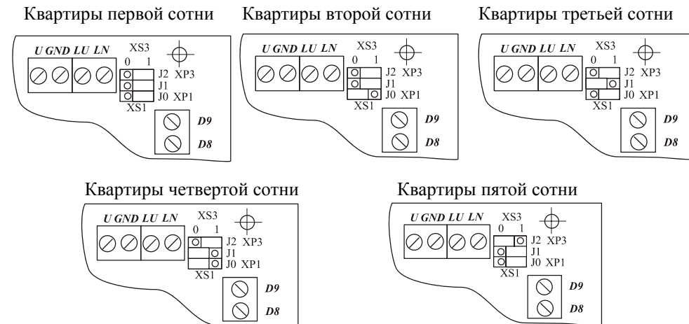
Рис.3 Положение джамперов XP1, XP2, и XP3 для различного диапазона квартир.
