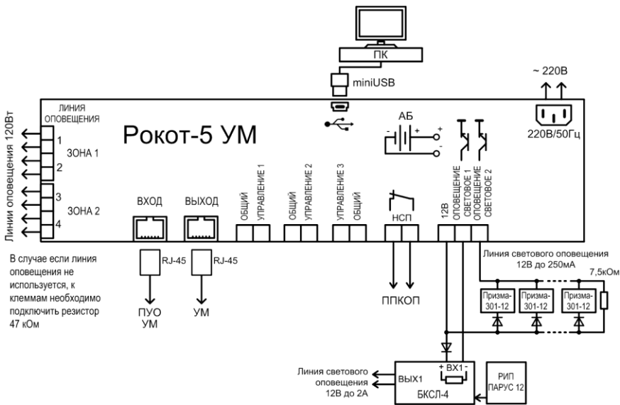
Рис.6 Схема внешних подключений «Рокот-5 УМ»
