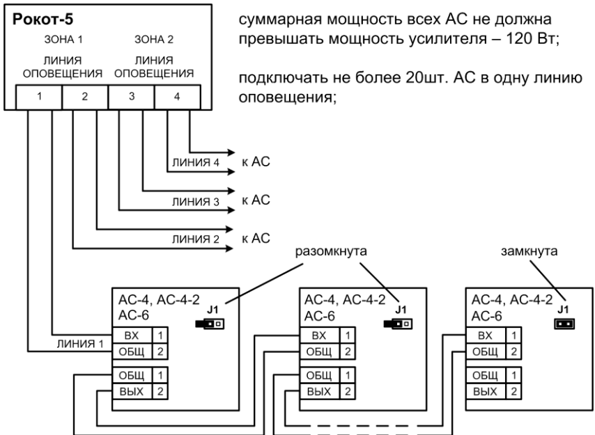
Рис.5а Схема подключений AC-4, AC-4-2, AC-6 к линиям оповещения
