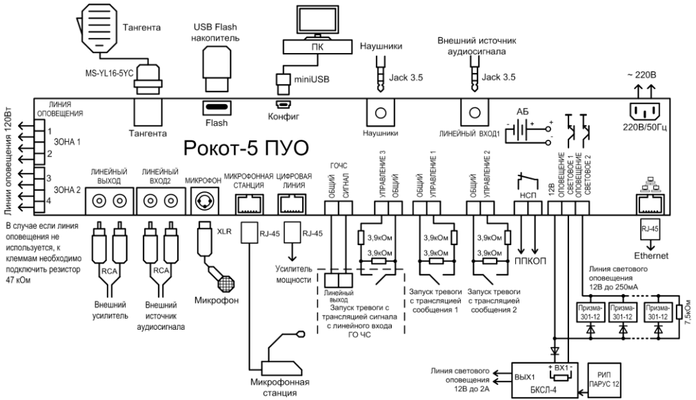
Рис.4 Схема внешних подключений «Рокот-5 ПДУ»
