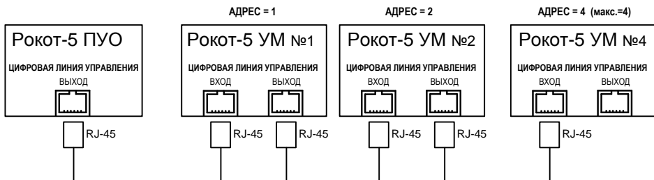
Рис.7 Схема соединения «Рокот-5 ПУО» и «Рокот-5 УМ» (всего можно подключить до 4-х усилителей мощности)
