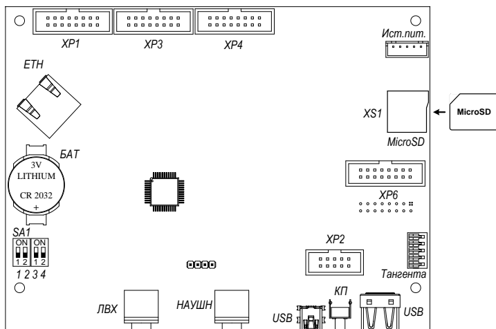
Рис.1 Внешний вид платы контроллера
