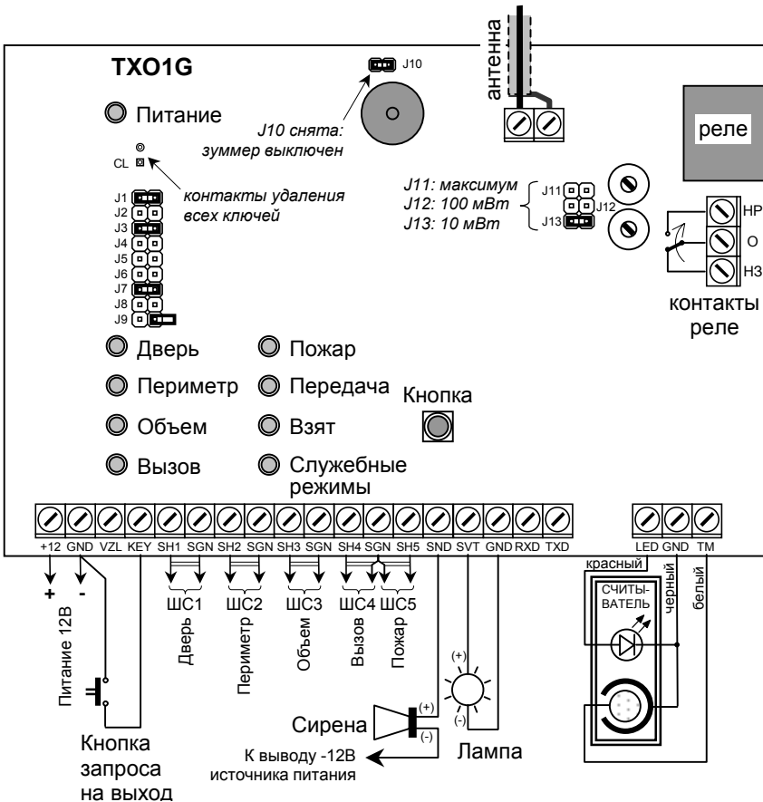
Рисунок 5 – Монтажная схема передатчика
