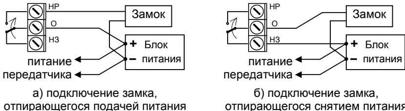
Рисунок 4 – Подключение электрического замка
