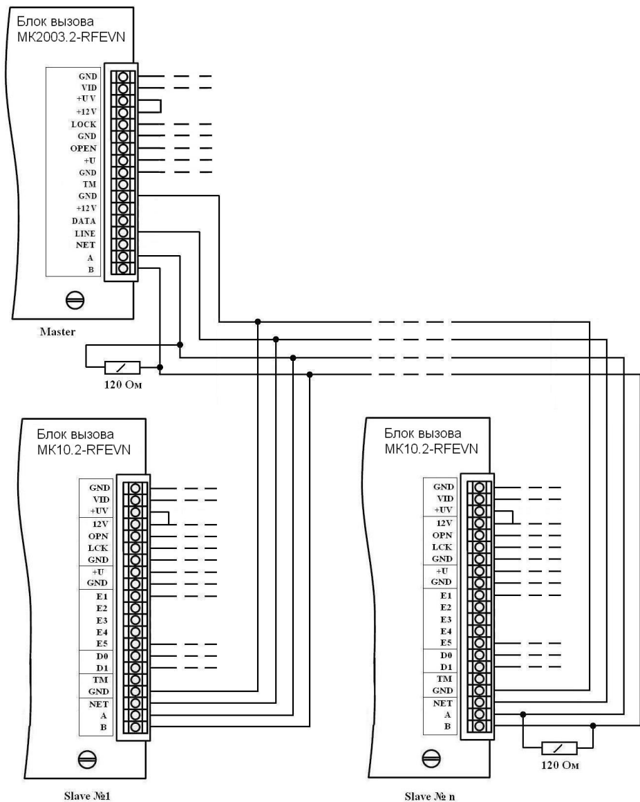
Рис. 3 Пример монтажа при объединении домофонов в сеть.
