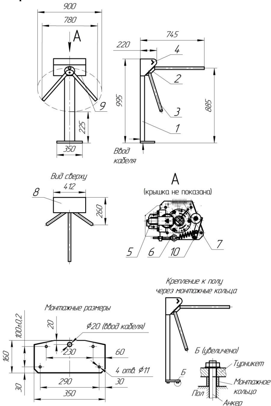
Габаритные и установочные размеры турникетов серии «Ростов-Дон Т9М1-02»
