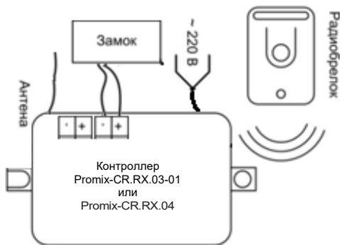
Рис.1.Блок-схема подключения комплекта
