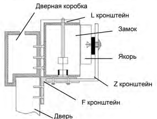
При помощи ZL кронштейна (BR-200ZL/BR-220L): (для дверей открывающихся наружу)
